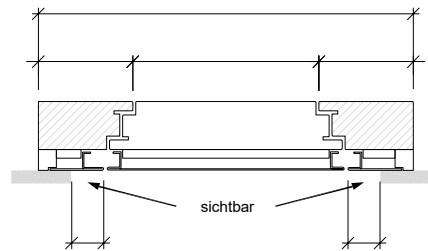
Ansschlagart Rahmen
