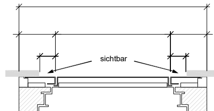
Anschlagart Rahmen
